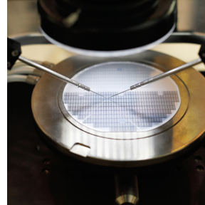
DUT
